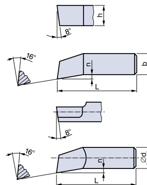
VNITŘNÍ UBÍRACÍ NŮŽ kód 223940 - pravý kód 223941 - levý
