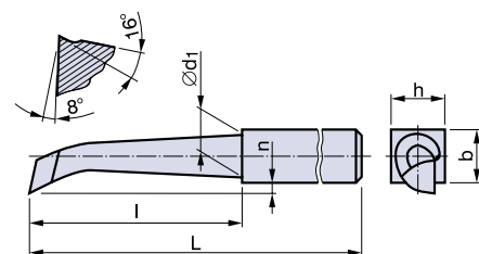
ZAPICHOVACÍ NŮŽ kód 223550 - pravý kód 223551 - levý
